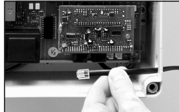
Коммуникационный провод протяните через изолятор
