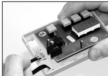
Коннектор защелкните в цоколь на плате пульта
